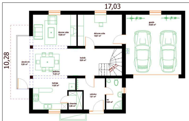
PRITLIČJE
