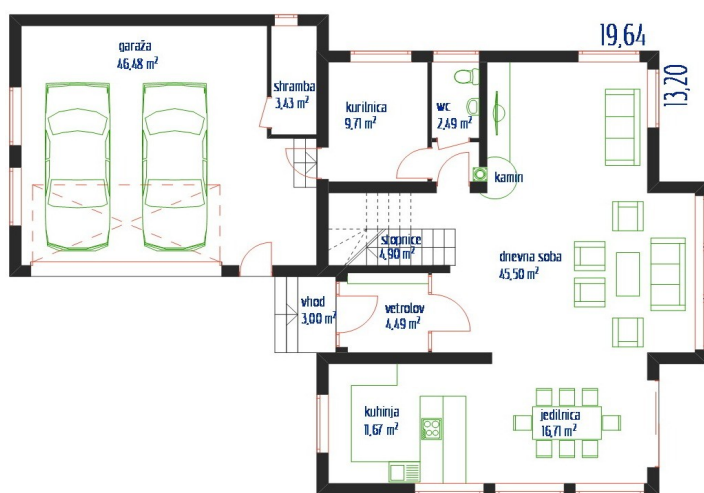
PRITLIČJE
